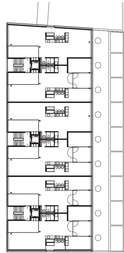
1.–5. Wohngeschoss
