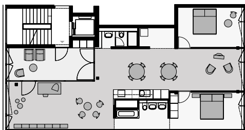
3-Raumwohnung, Wohngemeinschaft
