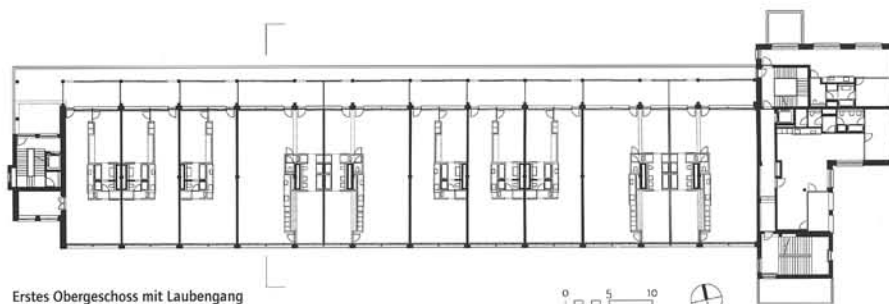
Erstes Obergeschoss mit Laubengang
