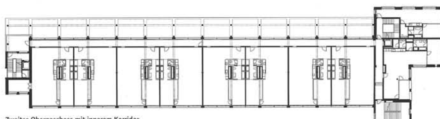
Zweites Obergeschoss mit innerem Korridor
