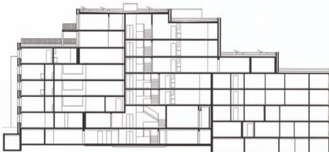
^ Längsschnitt: Das Treppenhaus im neuen Mittelteil verbindet die um ein halbes Geschoss versetzten Altbauten.
