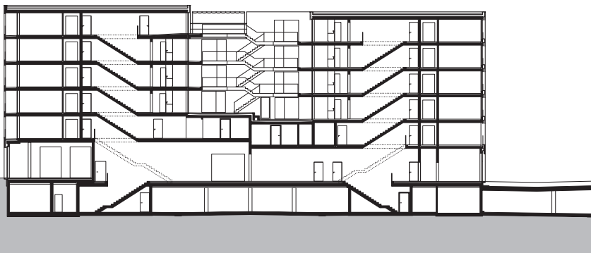
Längsschnitt
